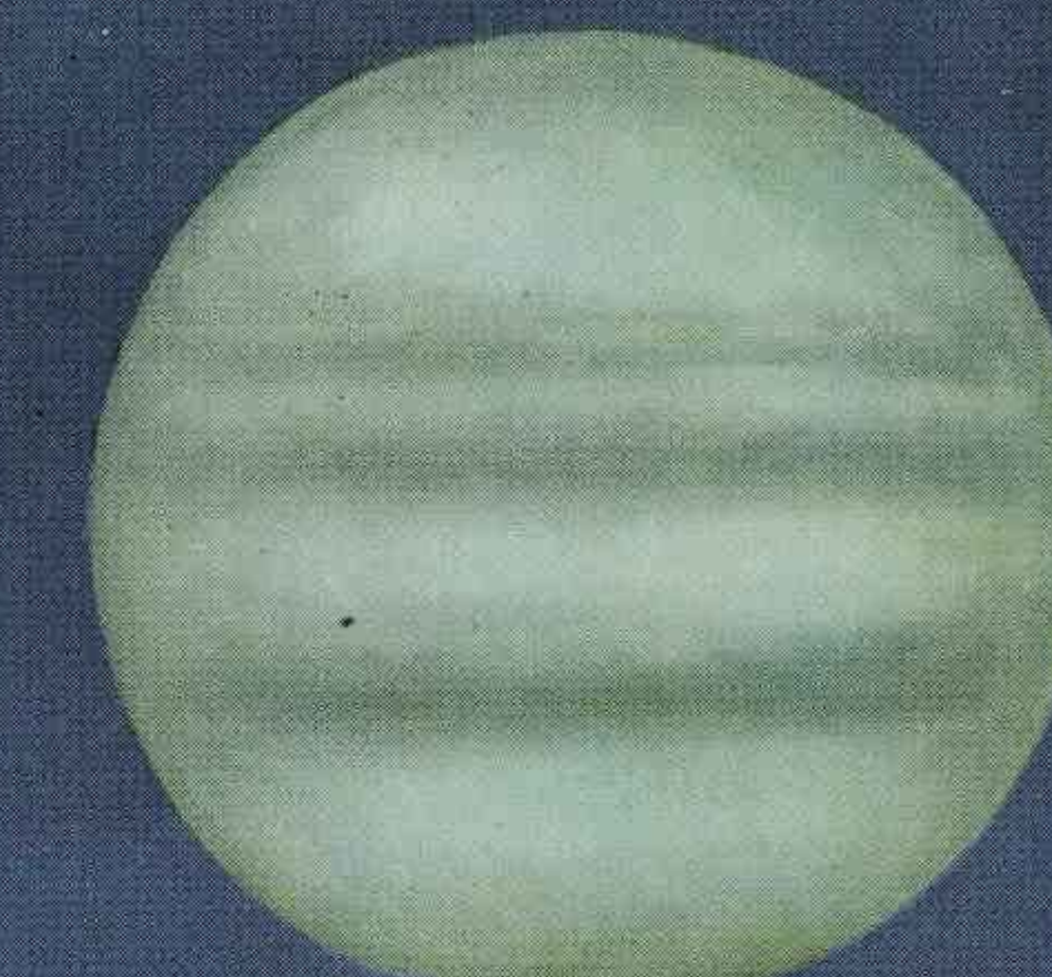
Neptuno
