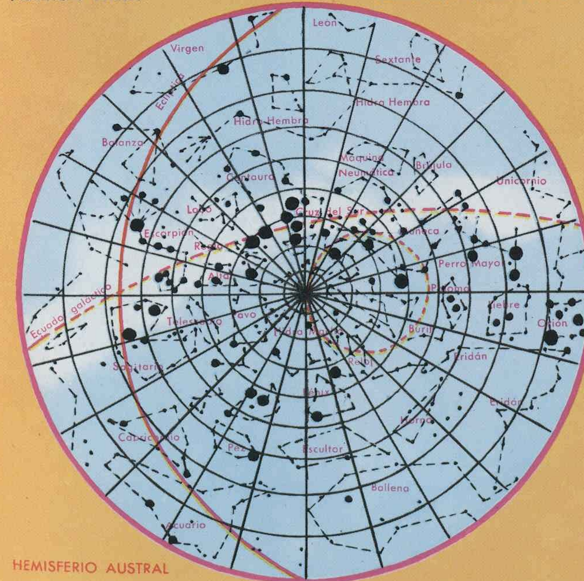
Planisferio celeste
