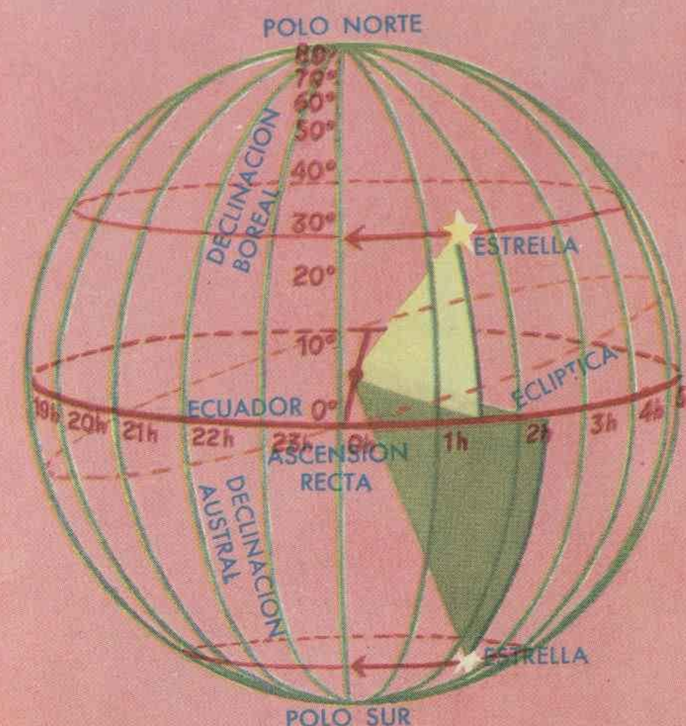
Coordenadas celestes.
