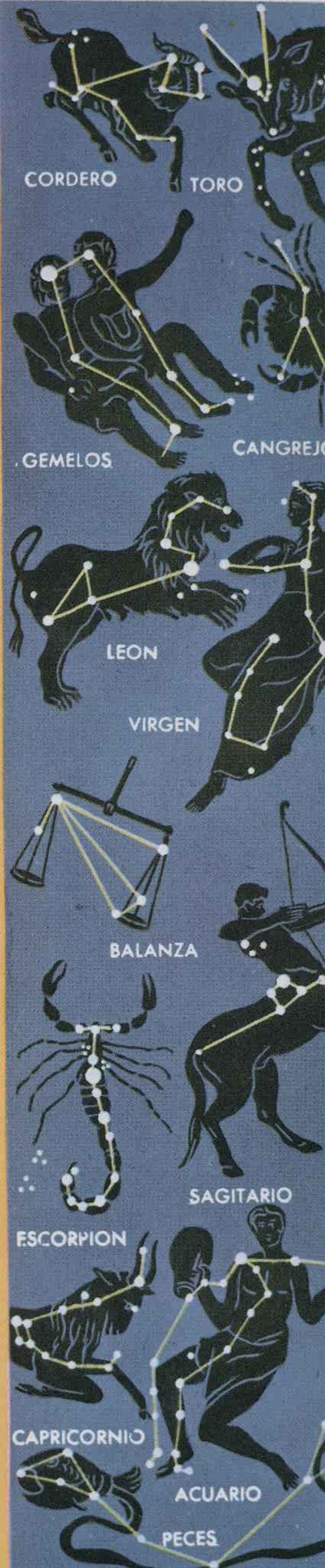
Constelaciones zodiacales →
